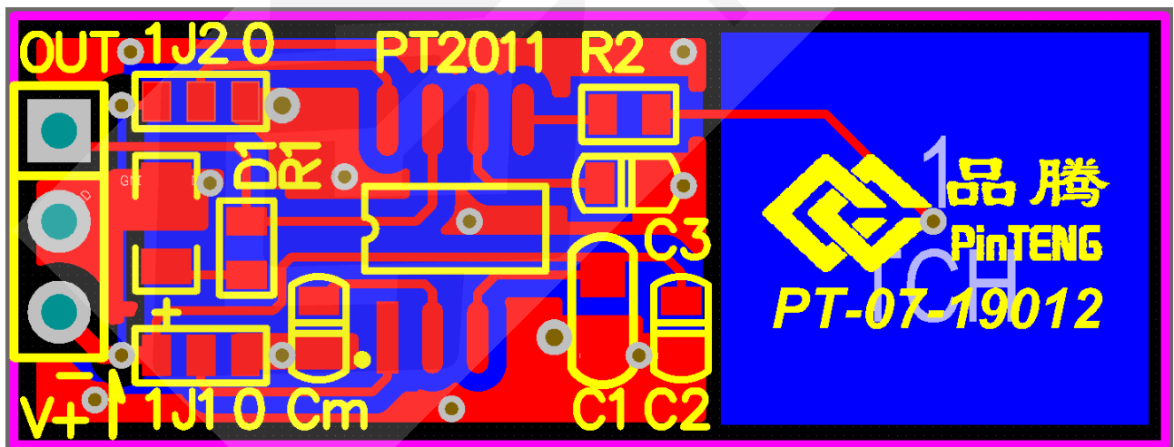
图 3 PCB 布线图
